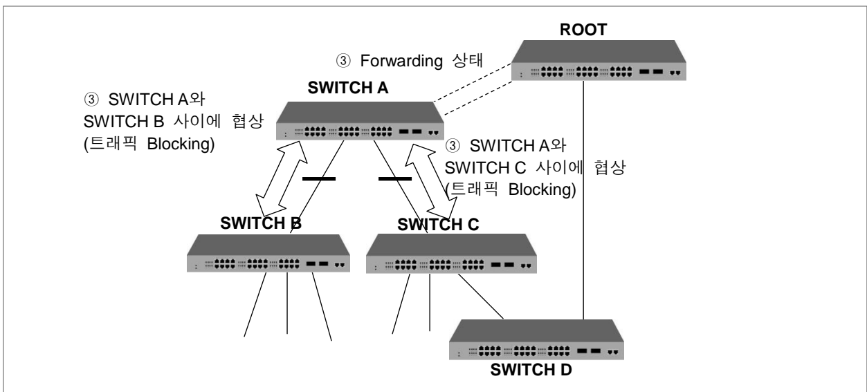
【 그림 8-22 】 802.1w의 네트워크 convergence ②
