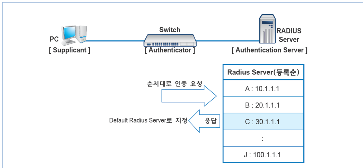
【 그림 4-2 】 Multi Authentication Server
