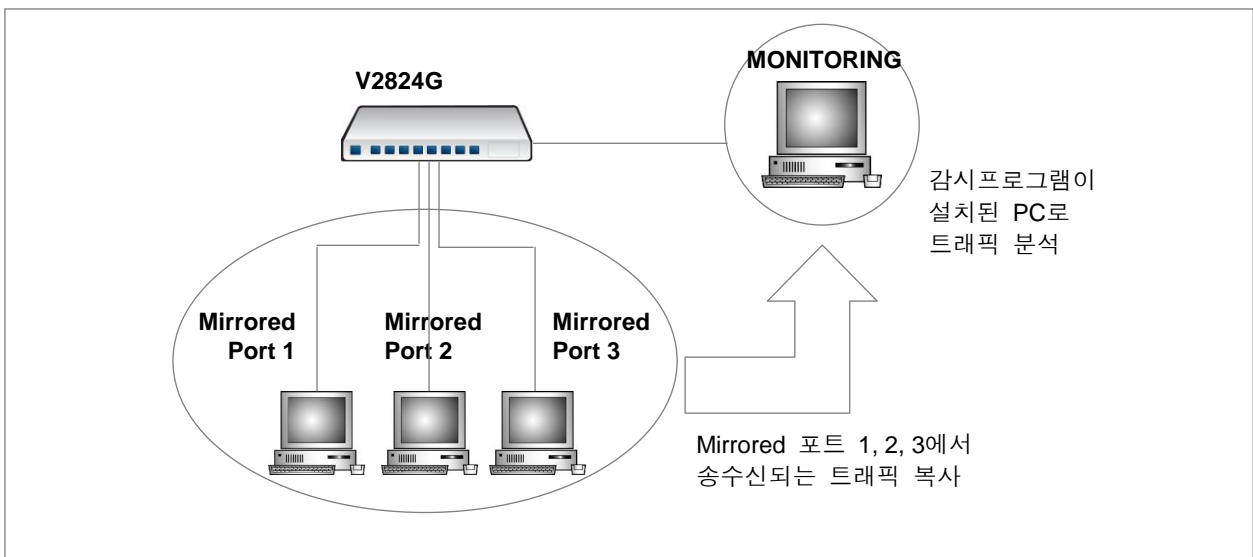
【 그림 5-1 】 포트 미러링의 예
