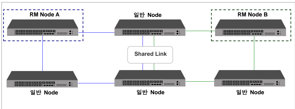
【 그림 8-35 】 Shared Link 환경
