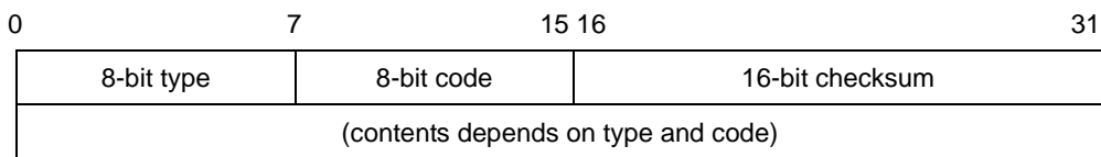
【 그림 7-15 】 ICMP 메시지
