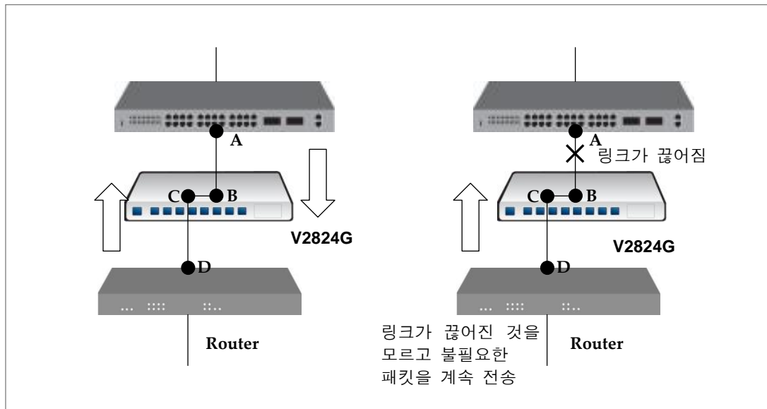
【 그림 7-17 】 LLCF 절차
