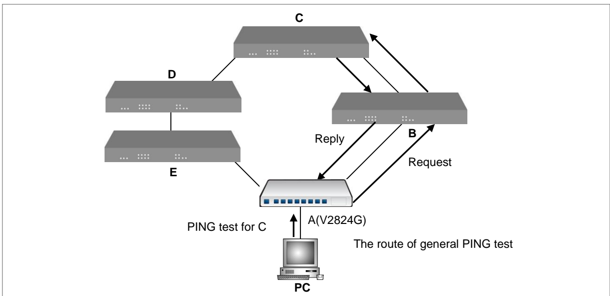
【 그림 6-2 】 네트워크 연결 확인을 위한 Ping 테스트
