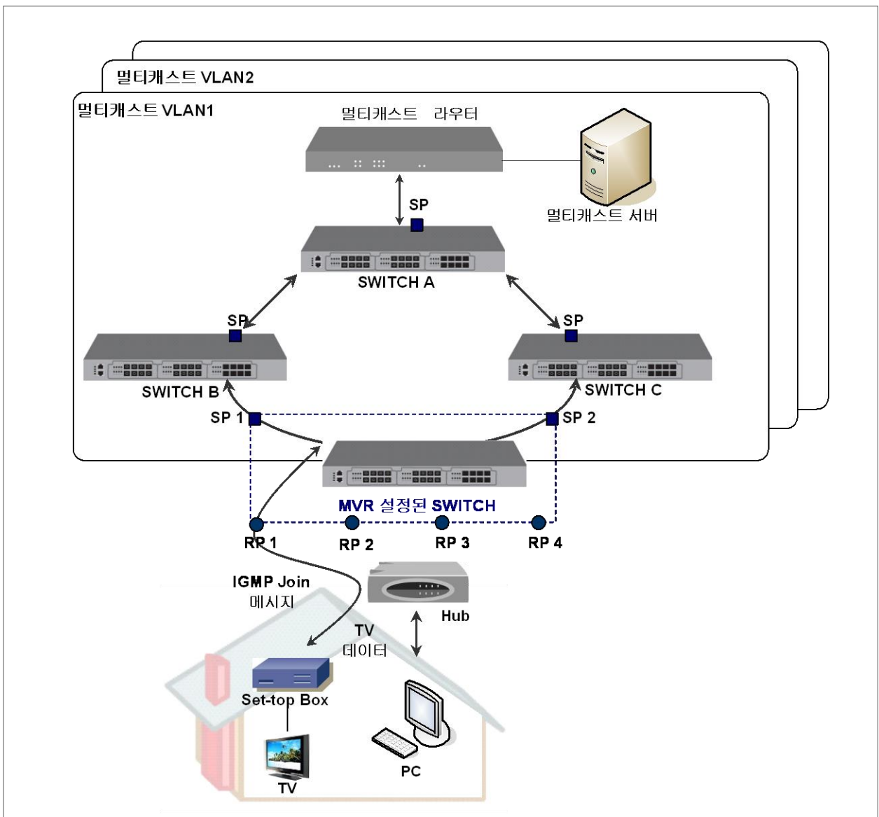
【 그림 9-6 】 MVR 동작
