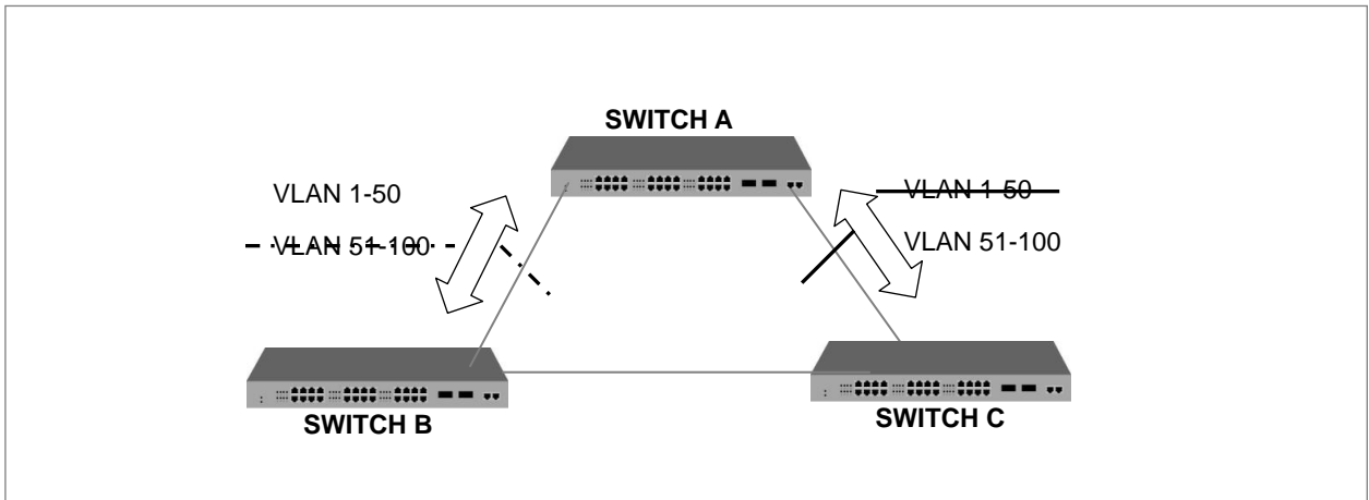
【 그림 8-27 】 PVSTP
