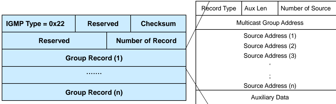
【 그림 9-4 】 IGMP 버전 3 Report 메시지 형식
