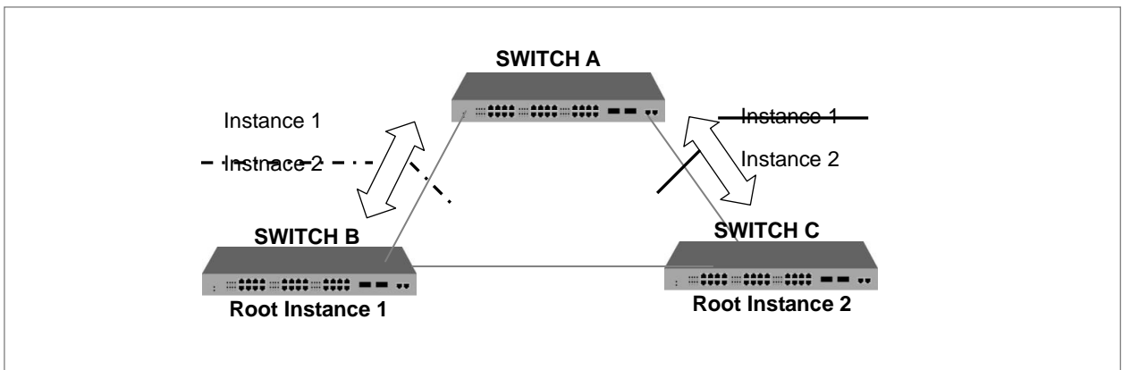
【 그림 8-28 】 MSTP
