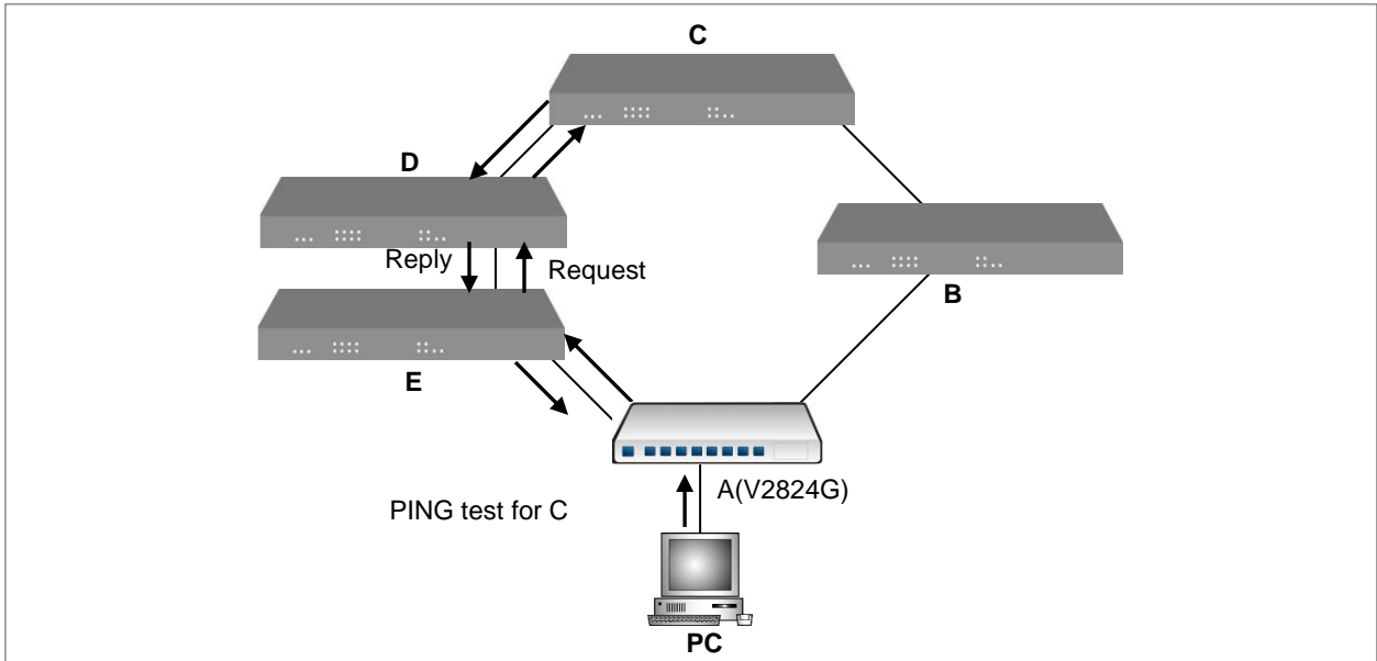
【 그림 6-3 】 IP ICMP Source Routing
