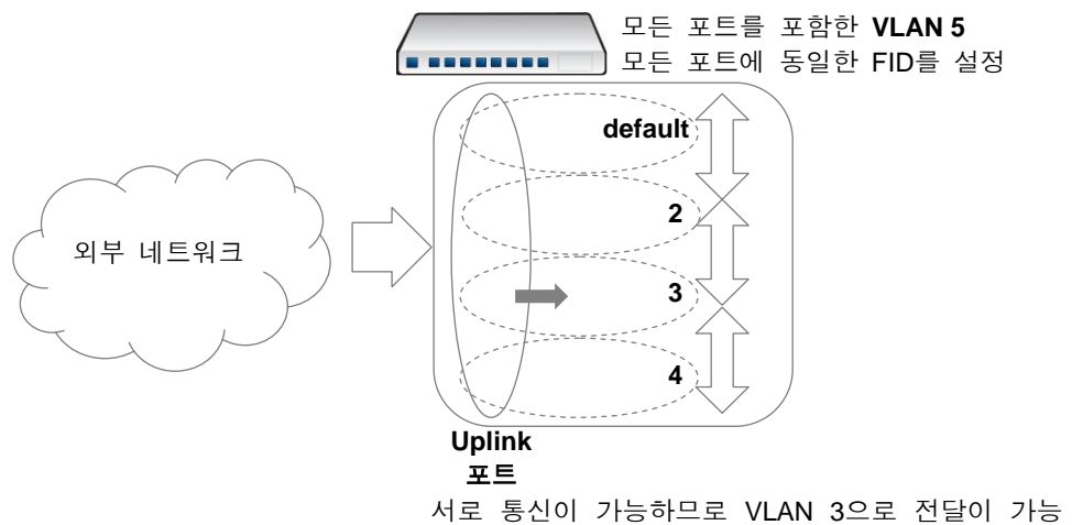
【 그림 8-7 】 Layer 2 환경에서 외부 패킷이 들어오는 경우 ②
