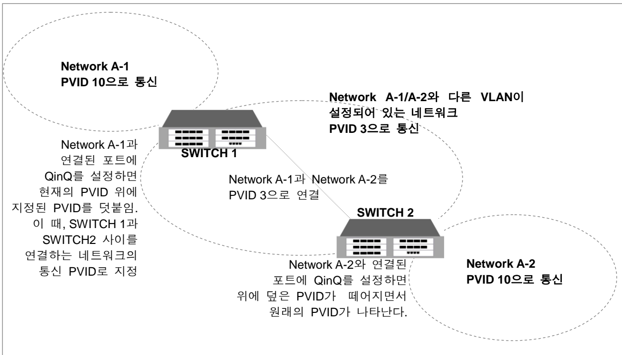
【 그림 8-4 】 QinQ 설정 네트워크 구성의 예
