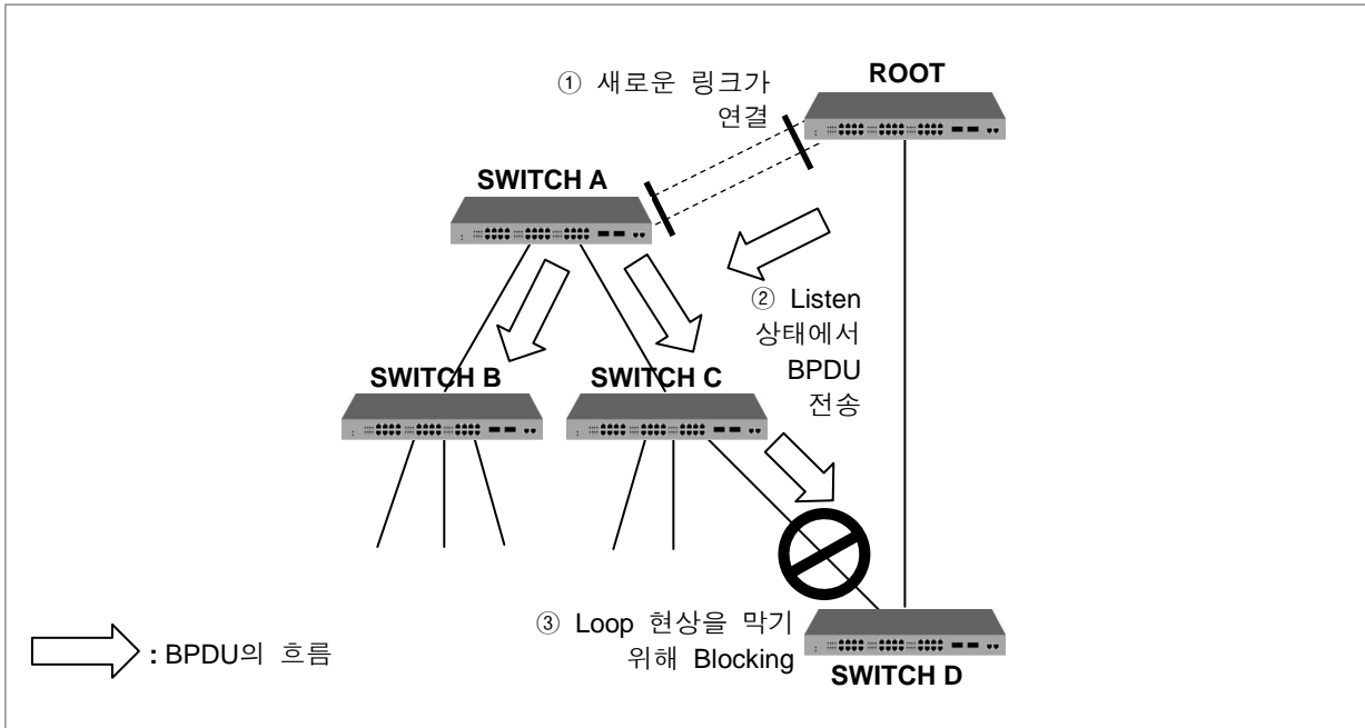
【 그림 8-20 】 802.1d의 네트워크 convergence
