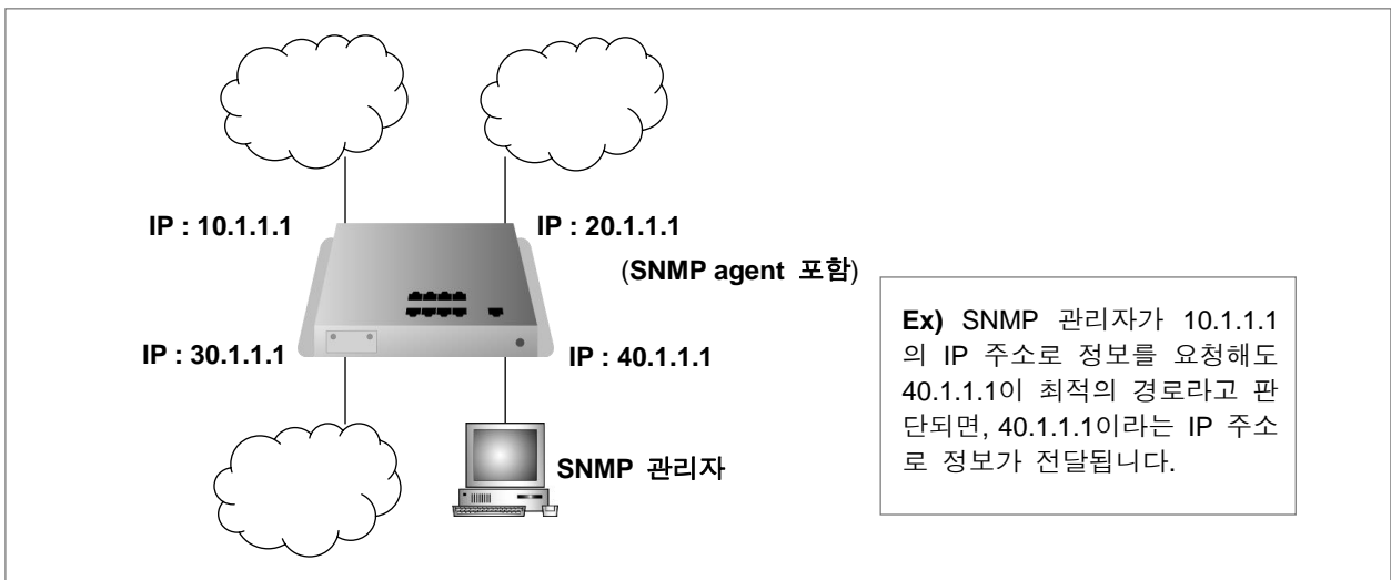
【 그림 7-2 】 SNMP 에이전트의 IP 주소
