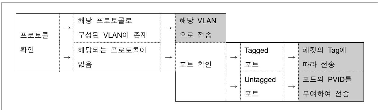
【 그림 8-3 】 VLAN 기준 패킷 경로 결정 절차
