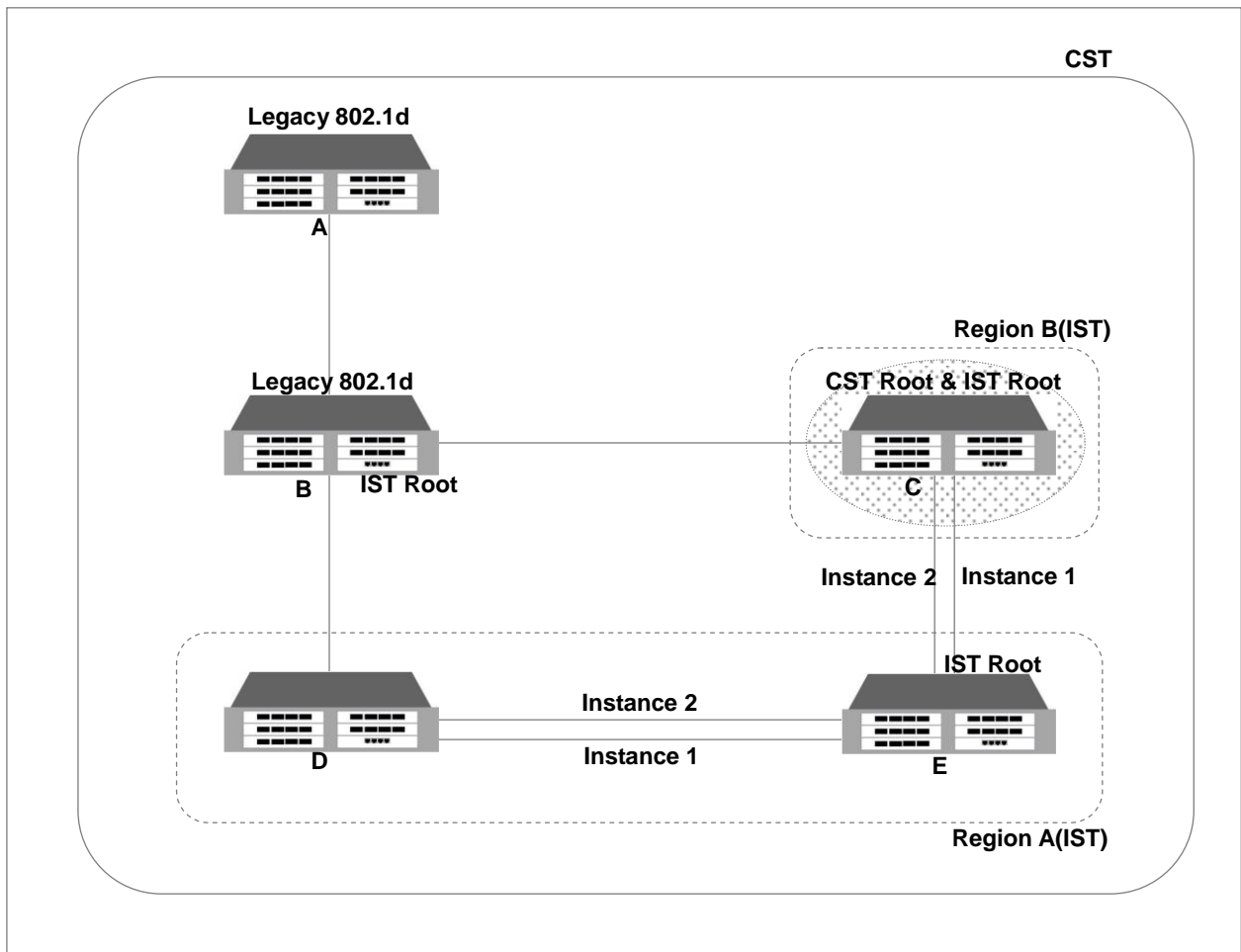
【 그림 8-29 】 MSTP의 CST와 IST①
