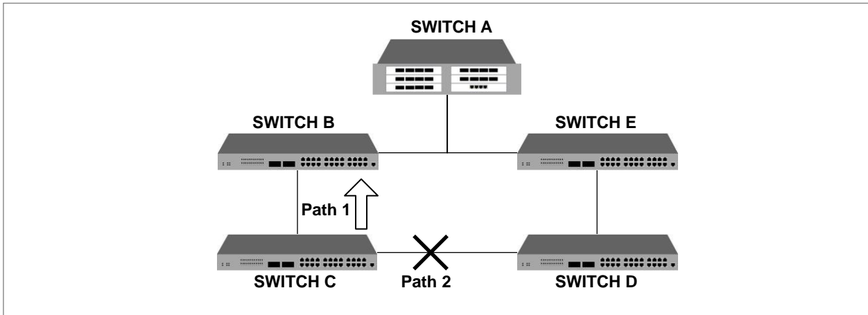
【 그림 8-13 】 STP의 원리
