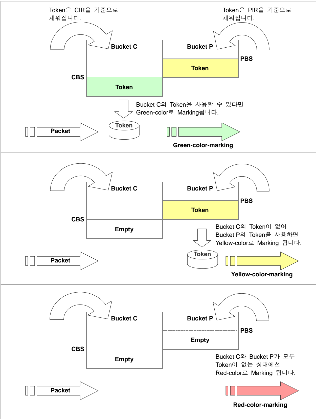
【 그림 7-8 】 Two Rate Three Color Marker의 Color Marking
