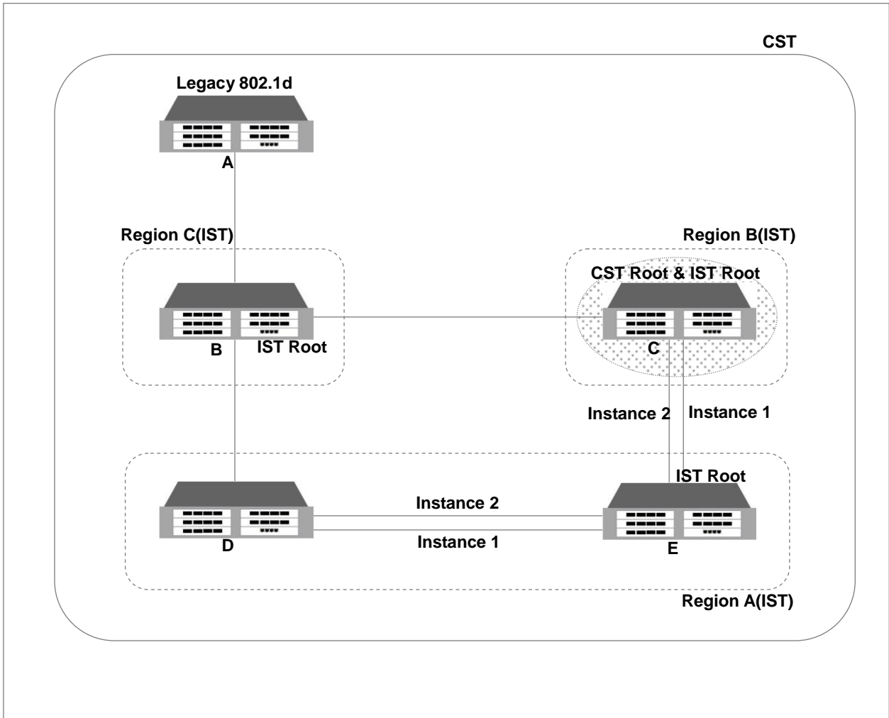
【 그림 8-30 】 MSTP의 CST와 IST②
