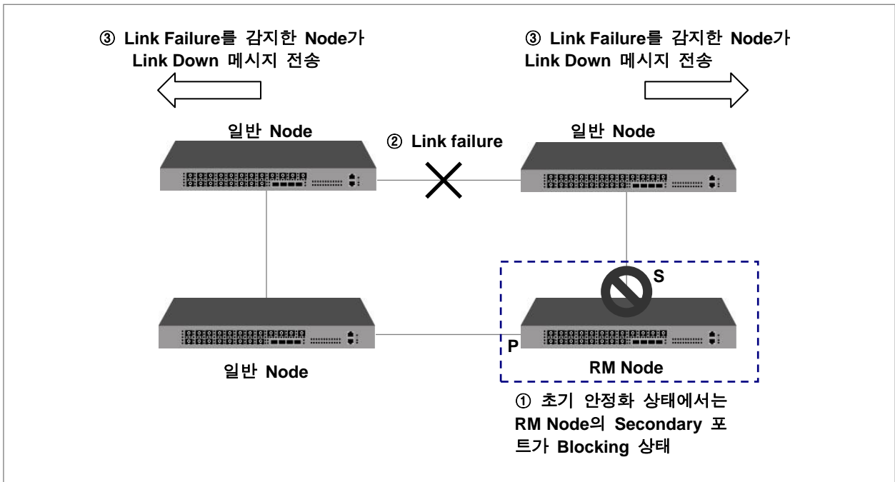
【 그림 8-31 】 Link failure 발생
