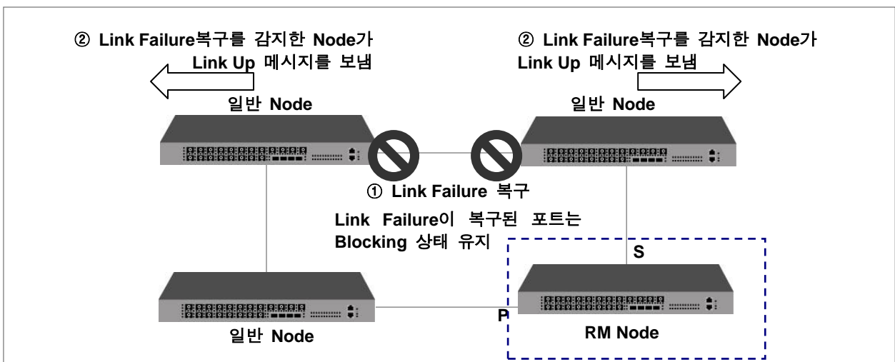
【 그림 8-33 】 Link Failure 복구
