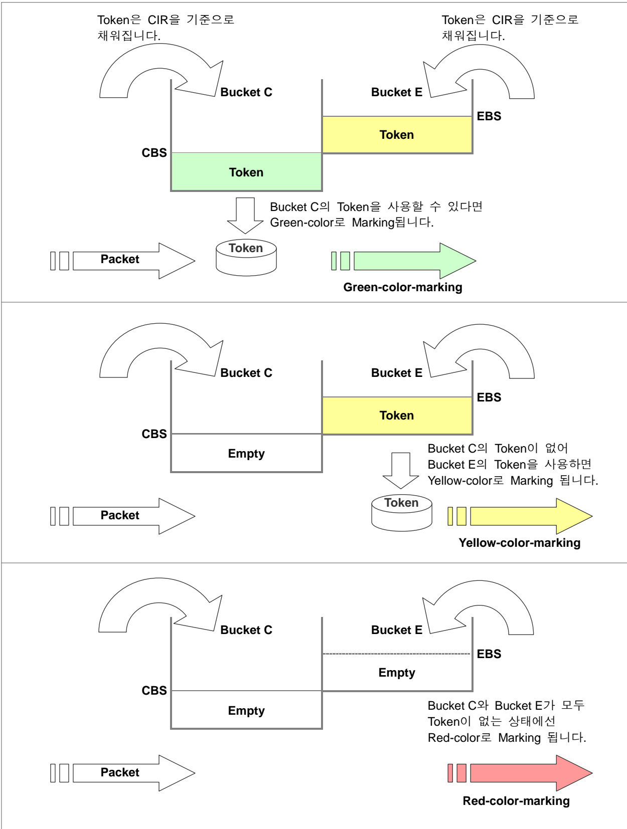
【 그림 7-7 】 Single Rate Three Color Marker의 Color Marking
