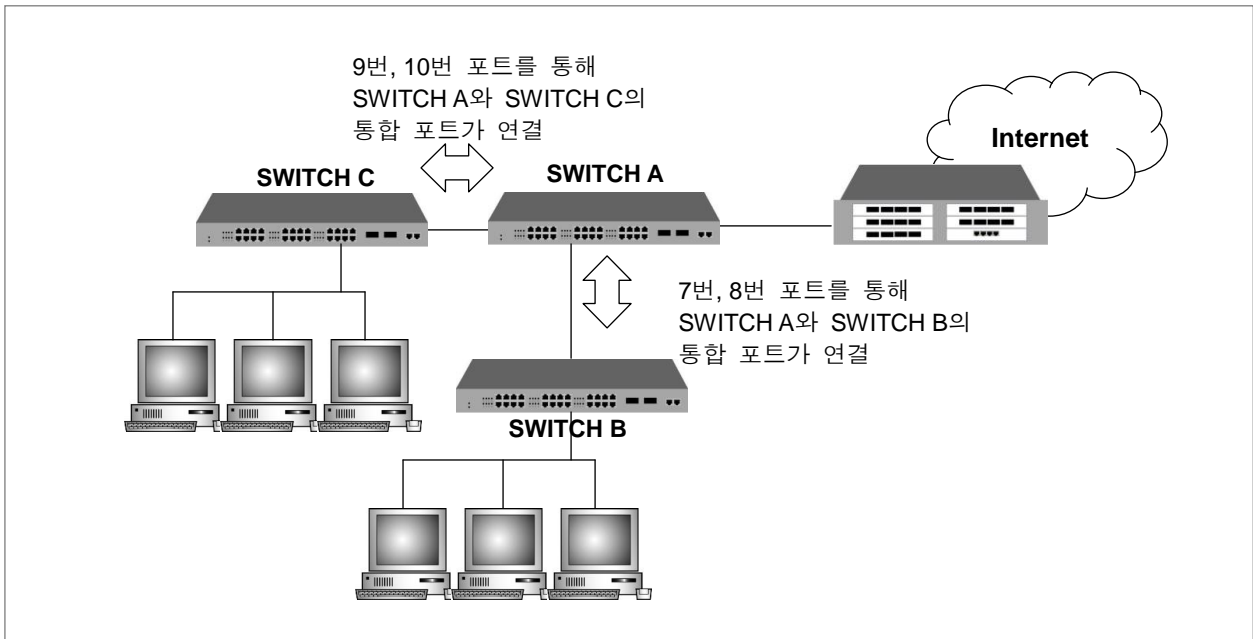
【 그림 8-10 】 LACP의 구성예 ①
