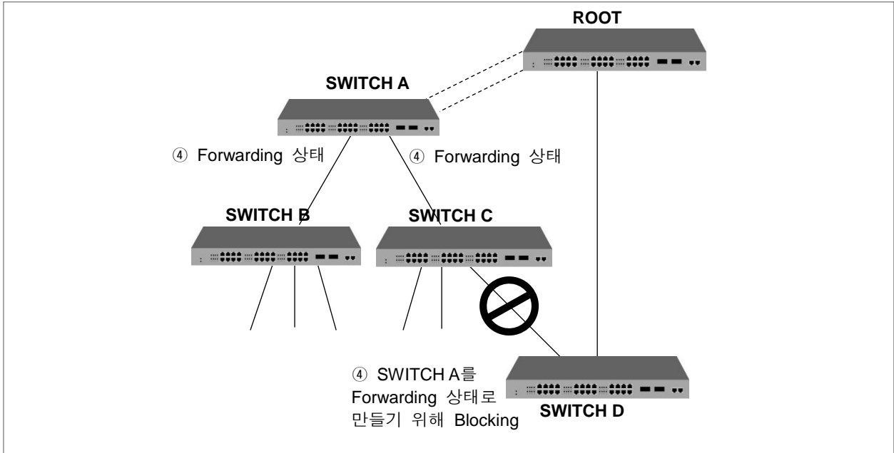
【 그림 8-23 】 802.1w의 네트워크 convergence ③
