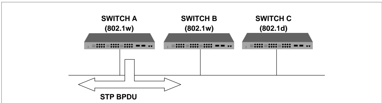
【 그림 8-25 】 STP와의 호환 ②
