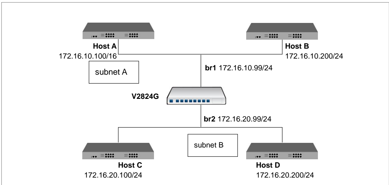
【 그림 7-14 】 Proxy-ARP
