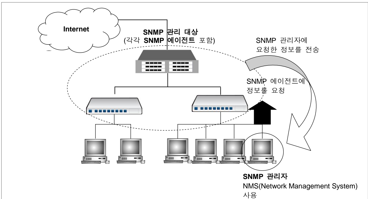
【 그림 7-1 】 SNMP 구성의 예
