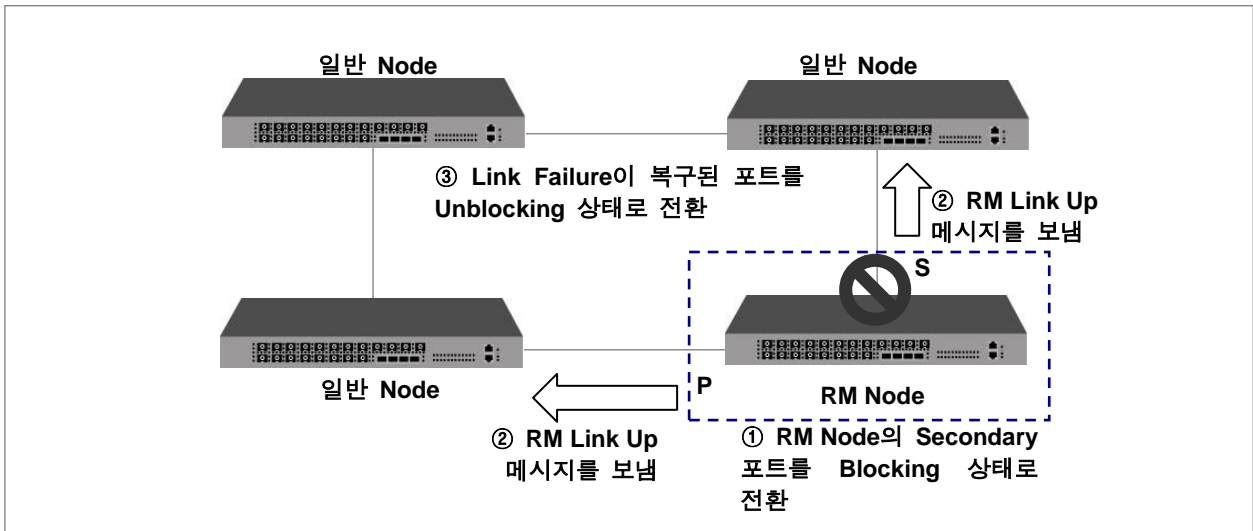
【 그림 8-34 】 Ring Recovery
