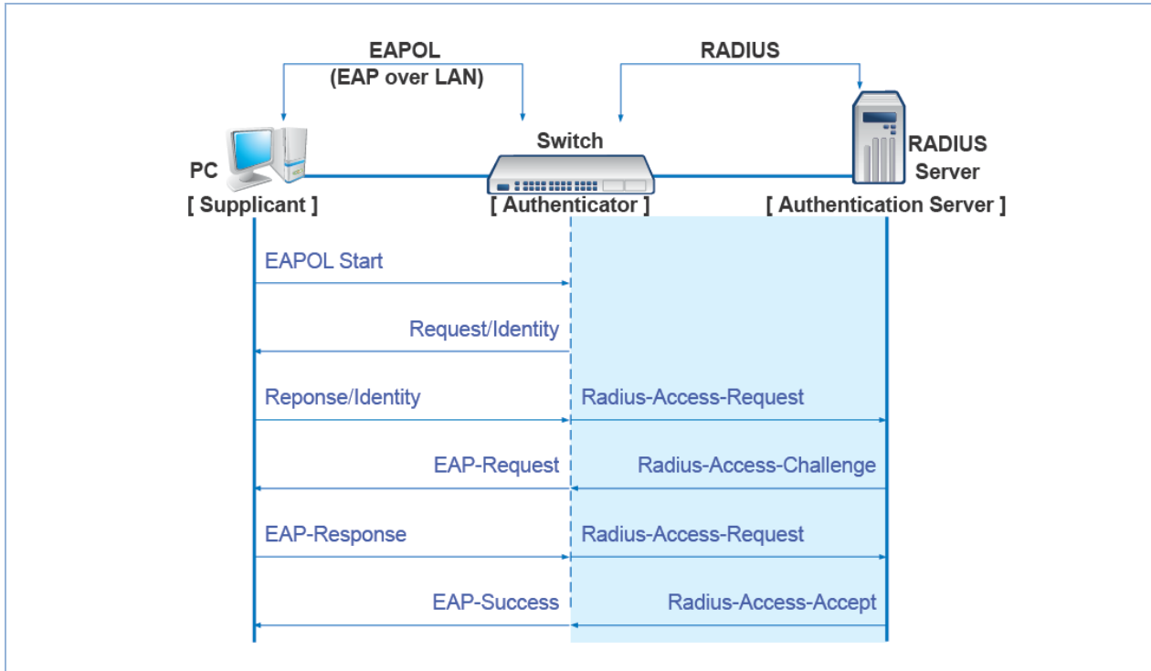
【 그림 4-1 】 802.1x 사용자 인증 과정
