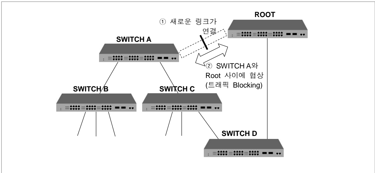
【 그림 8-21 】 802.1w의 네트워크 convergence ①
