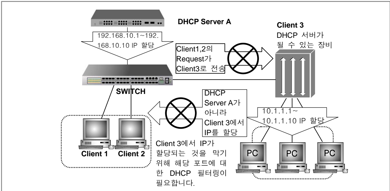
【 그림 7-13 】 DHCP 필터링
