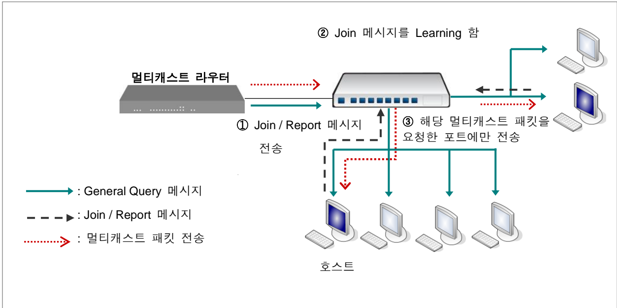
【 그림 9-5 】 IGMP Snooping을 설정했을 경우
