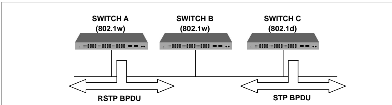
【 그림 8-24 】 STP와의 호환 ①
