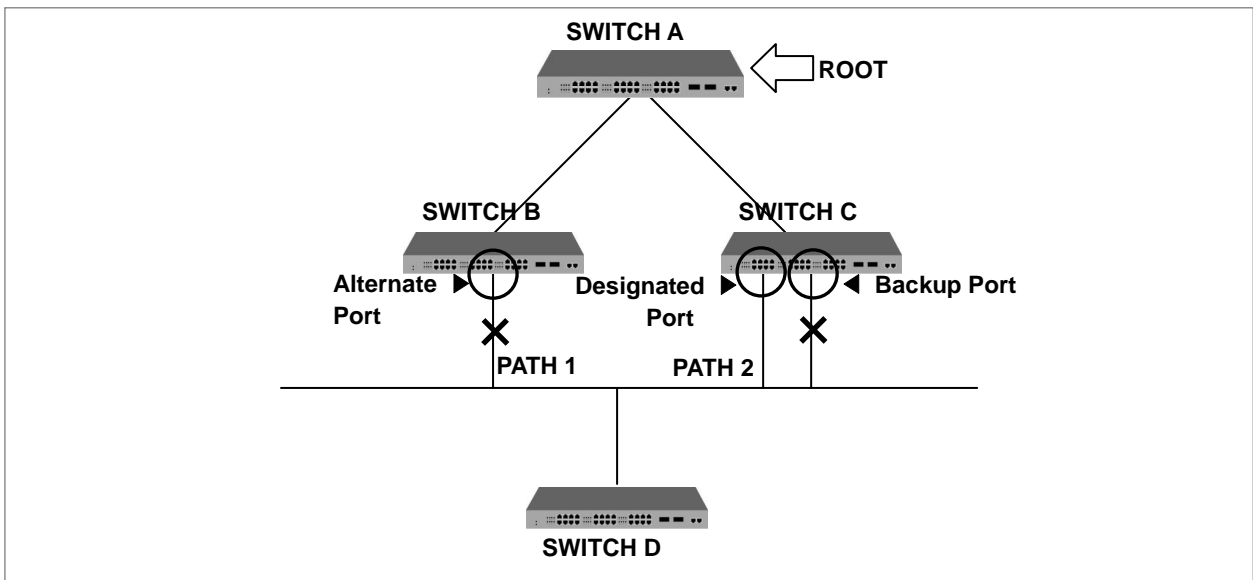
【 그림 8-18 】 Alternate 포트와 Backup 포트
