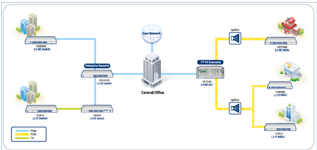
【 그림 2-1 】 V2824G를 이용한 네트워크 구성의 예
