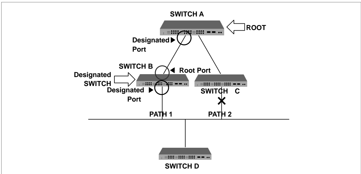
【 그림 8-16 】 Designated 스위치와 Designated 포트
