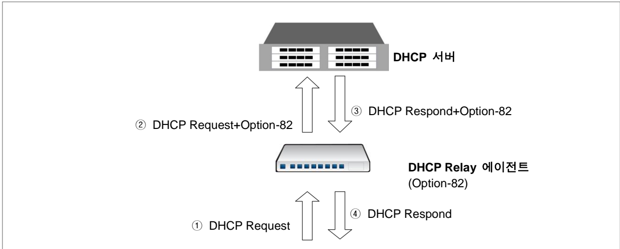
【 그림 8-40 】 DHCP Option-82를 사용하는 경우의 패킷 흐름
