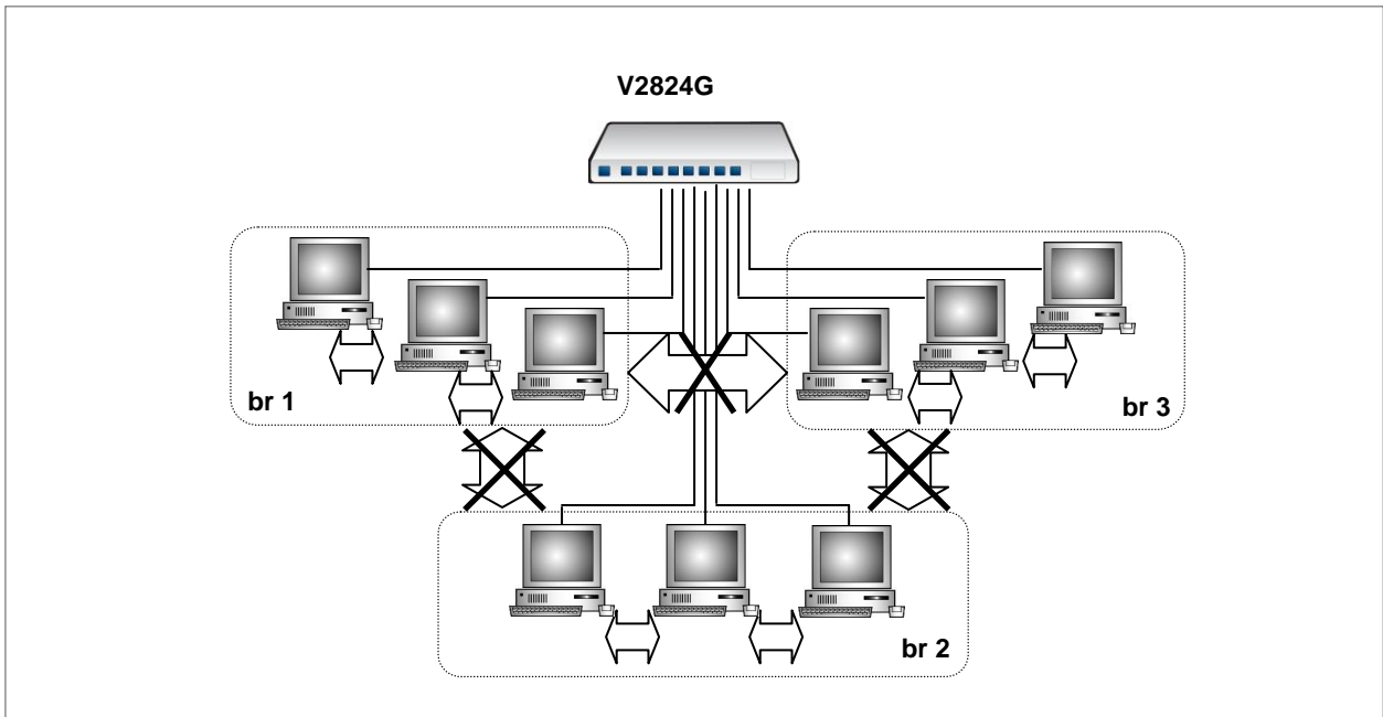
【 그림 8-2 】 Layer 2 환경 포트 기준 VLAN 구성도
