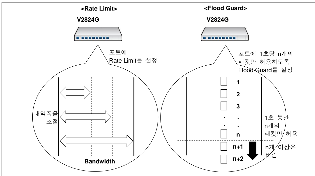
【 그림 8-37 】 Rate Limit와 Flood Guard
