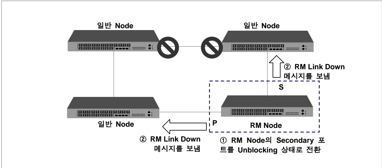
【 그림 8-32 】 Ring Protection
