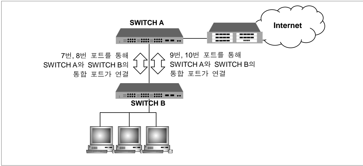
【 그림 8-11 】 LACP의 구성예 ②
