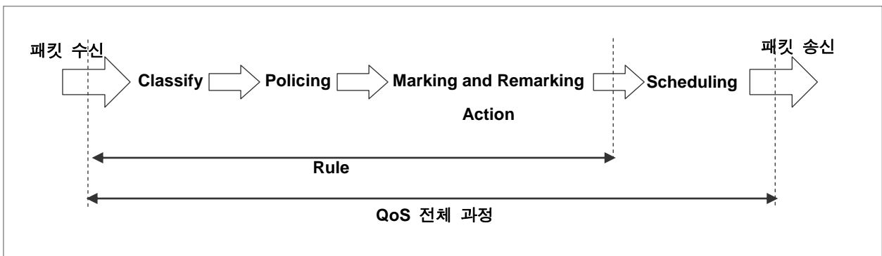
【 그림 7-4 】 QoS의 동작 구조
