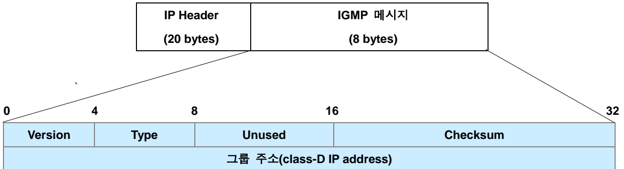
【 그림 9-1 】 IGMP 버전 1 메시지 형식
