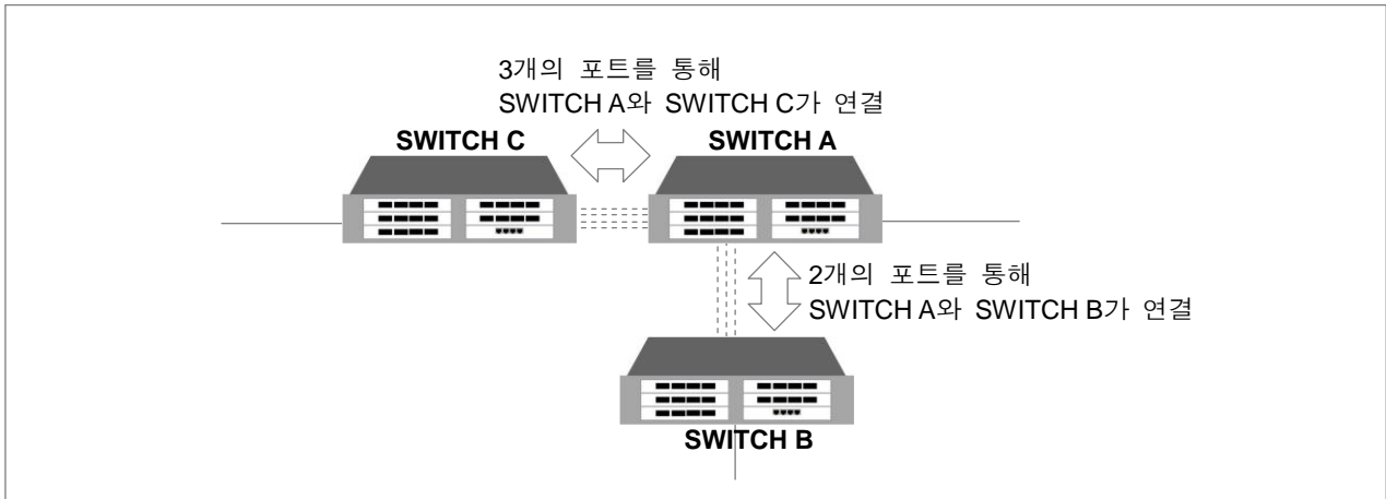
【 그림 8-9 】 Link Aggregation 구성예 ①
