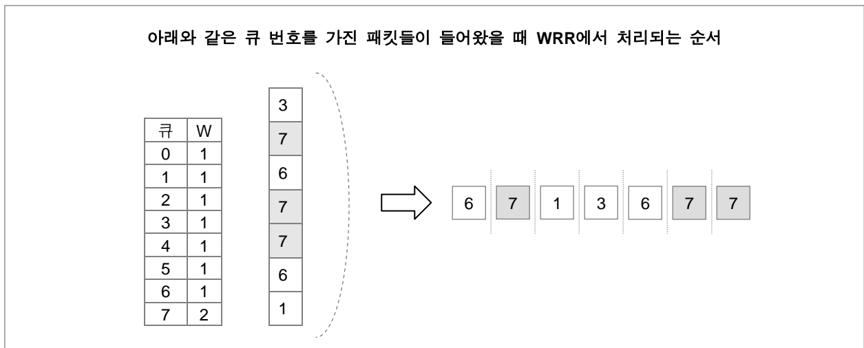
【 그림 7-10 】 WRR에서의 패킷 처리
