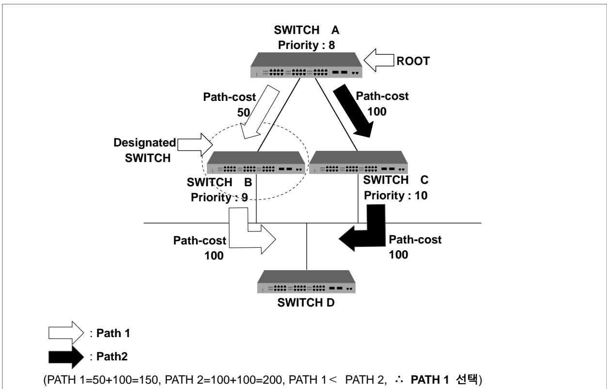
【 그림 8-15 】 Designated 스위치 결정
