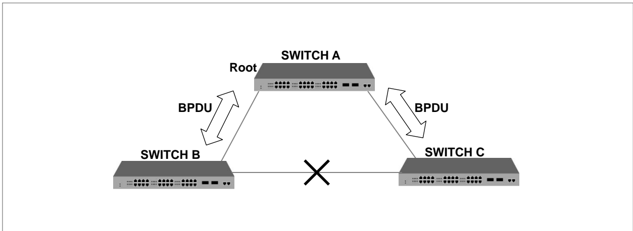
【 그림 8-26 】 STP
