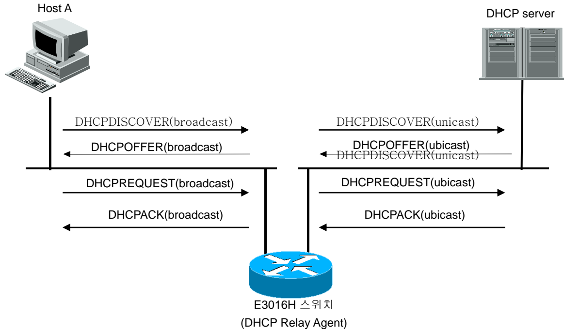
그림 1. DHCP Relay Agent 로서 DHCP Server 의 메시지 전달
