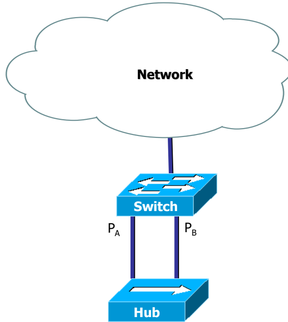
그림 4 self-loop 발생 환경 2
