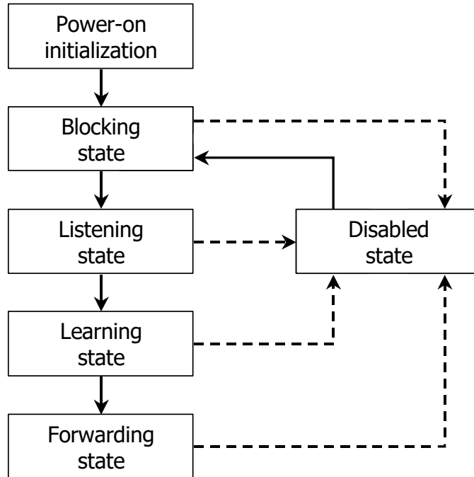
그림 2 Spanning-Tree Interface States
