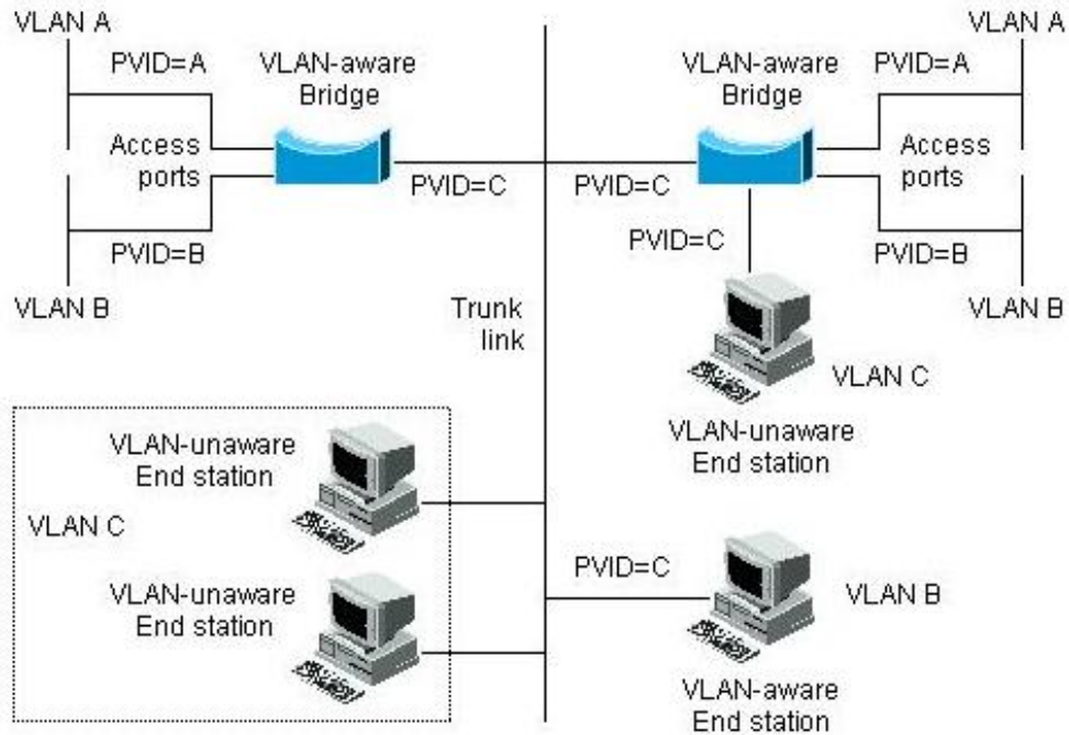
그림 6. Native VLAN
