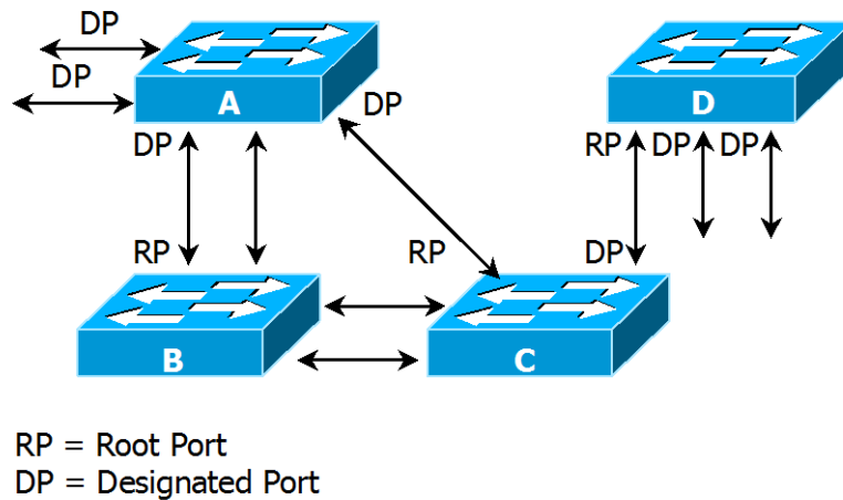
그림 1 Spanning-Tree Topology
