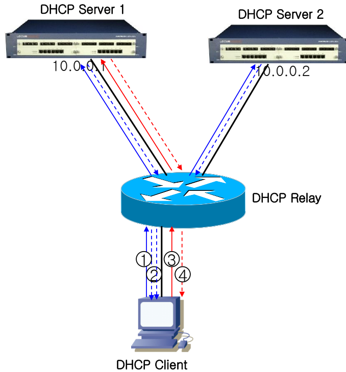
그림 4. DHCP Relay Server-Id-Relay 동작 절차
