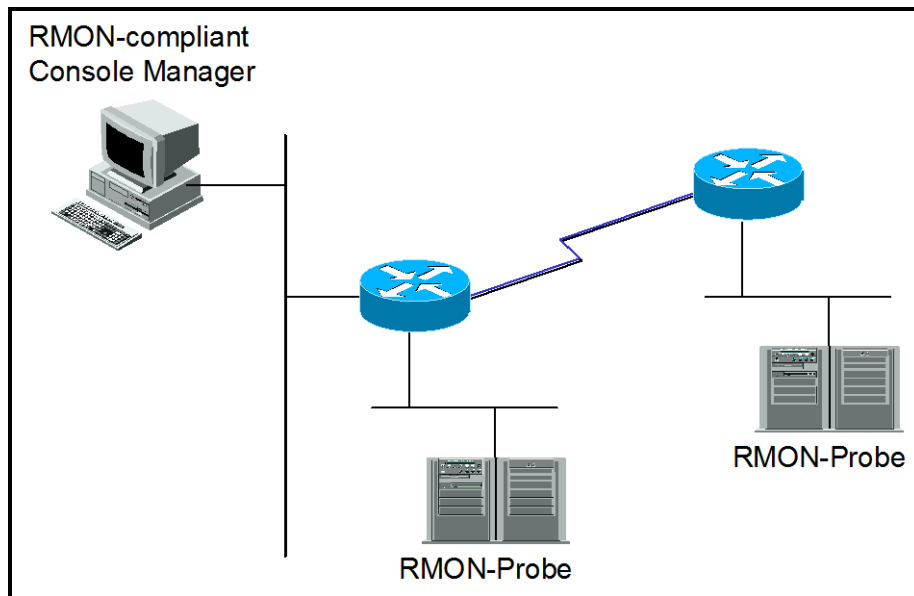
■ 그림 1. RMON Manager와 RMON Probe
