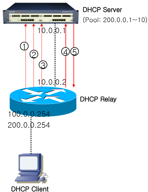
그림 3. DHCP Smart-Relay 동작 절차
