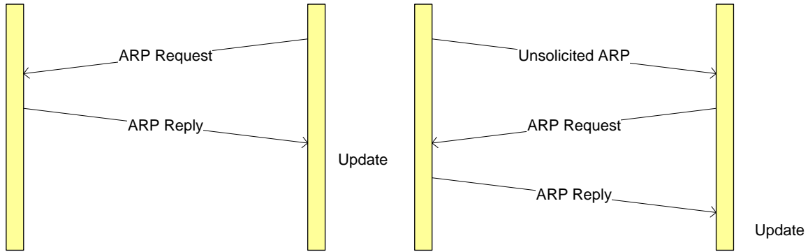
그림 1 ARP snoop (3-way handshake)
