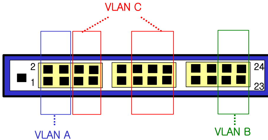
그림 1. E3016H Series 스위치의 포트 기반 VLAN 구성 예
