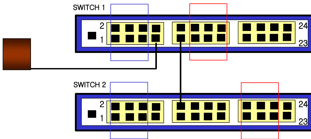
그림 4. 태그가 붙은 프레임과 태그가 붙지 않은 프레임의 물리적 다이어그램
