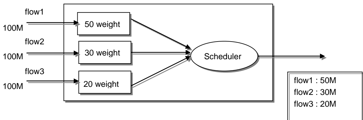
■ 그림 3. WRR Method
