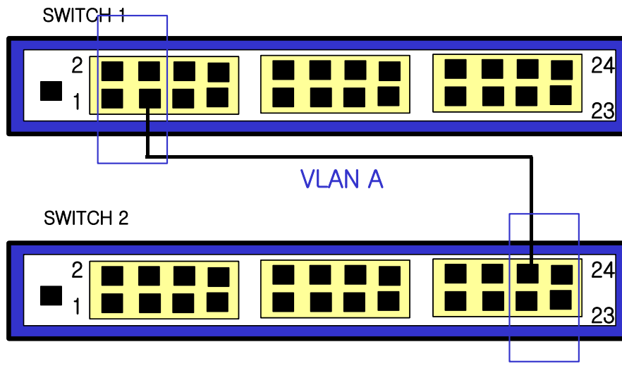
그림 2. 두 스위치에 걸쳐서 설정된 단일 포트 기반 VLAN
