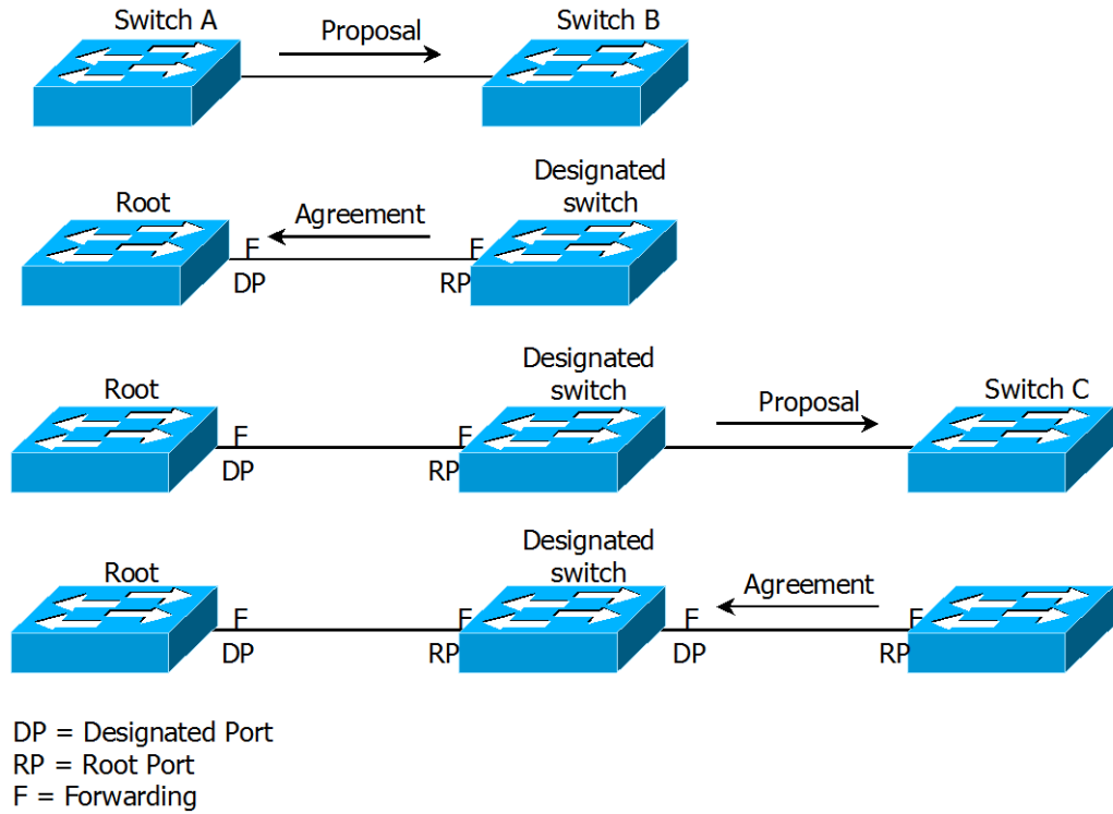
그림 3 Proposal and Agreement Handshaking for Rapid Convergence
