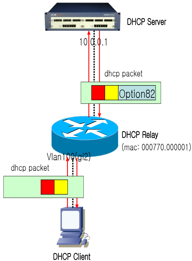
그림 2. DHCP Relay Option82
