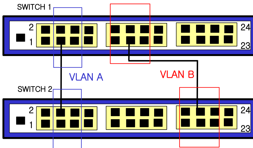
그림 3. 두 스위치에 걸쳐서 설정된 두 개의 포트 기반 VLAN
